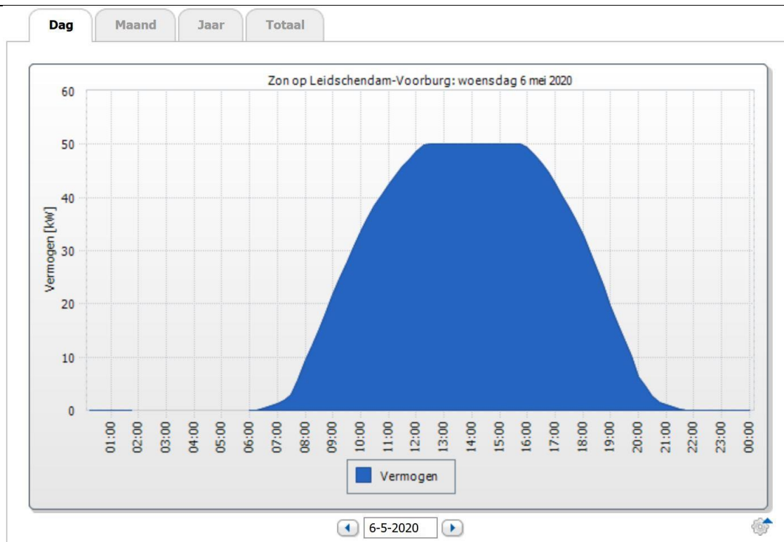
Afbeelding 2: Opbrengst 459 kWh..
